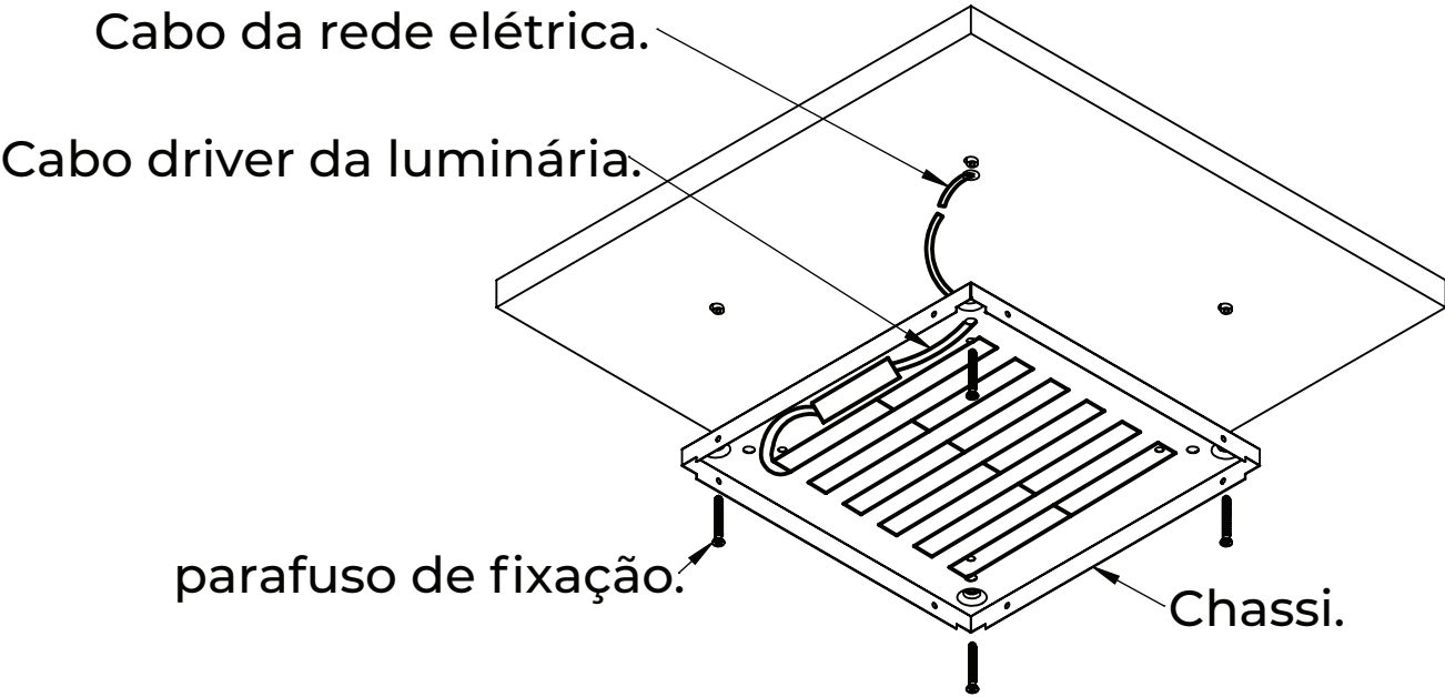
2. Fixe o chassi com parafuso e Conecte os cabos da rede elétrica.
