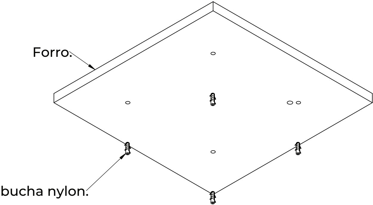
1. Fixe as buchas na superfície demarcada.
