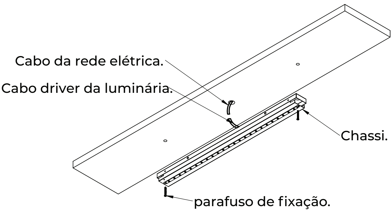
2. Fixe o chassi com parafuso e Conecte os cabos da rede elétrica.
