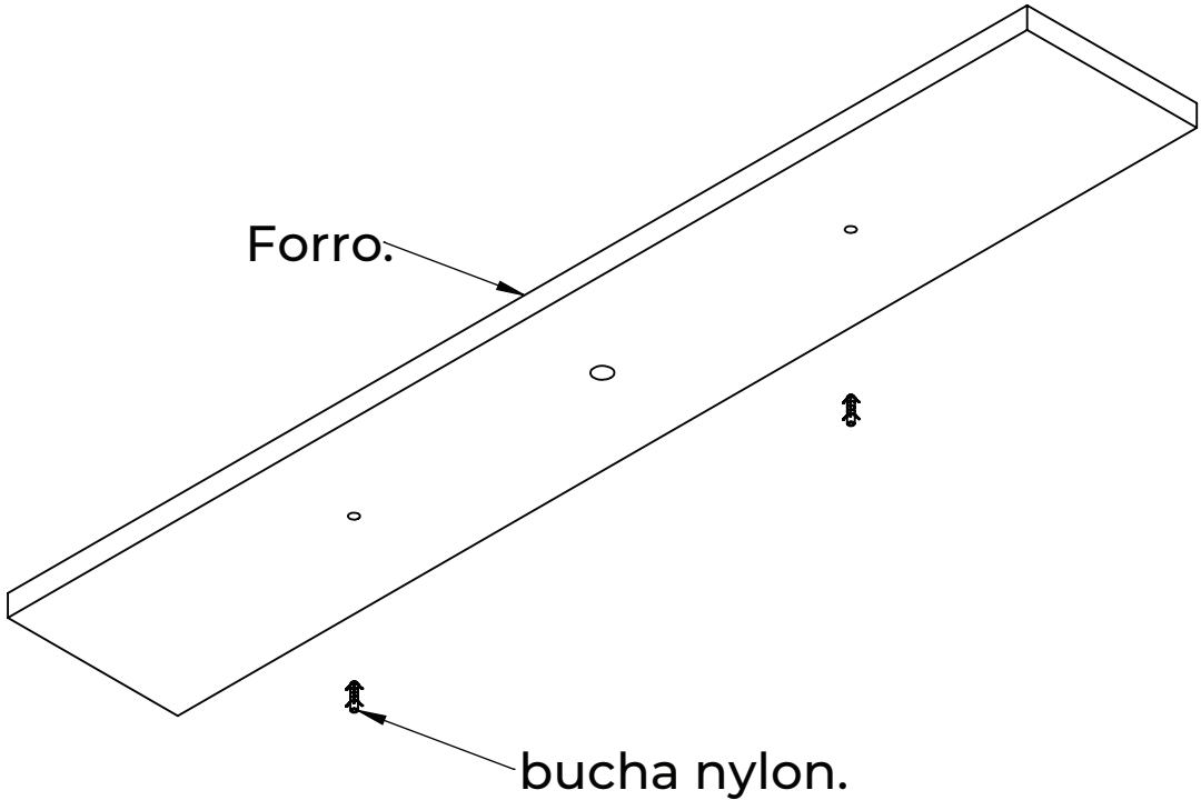
1. Fixe as buchas na superfície demarcada.
