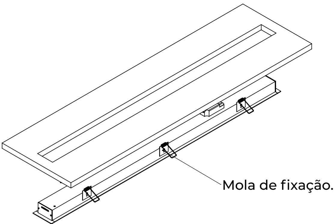
3. Suspenda a luminária fixando com as molas.
